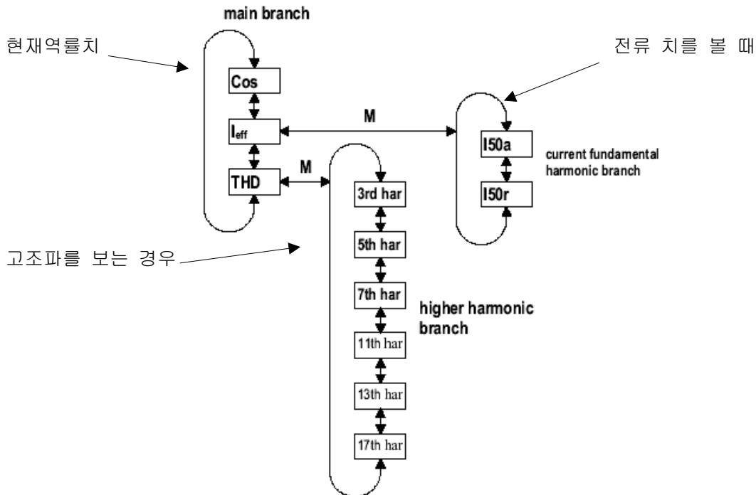
[그림2] 표시 부의 메인 흐름도
