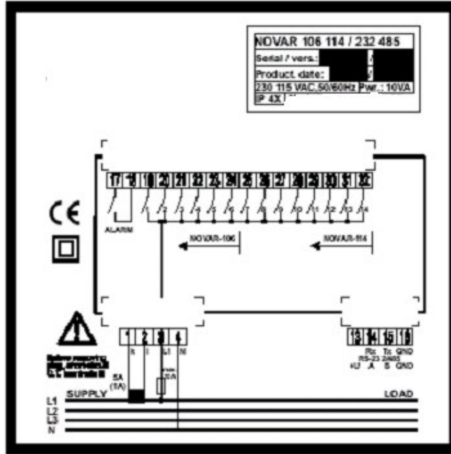
[그림3] novar 106,114의 경우 후면 단자 결선도
